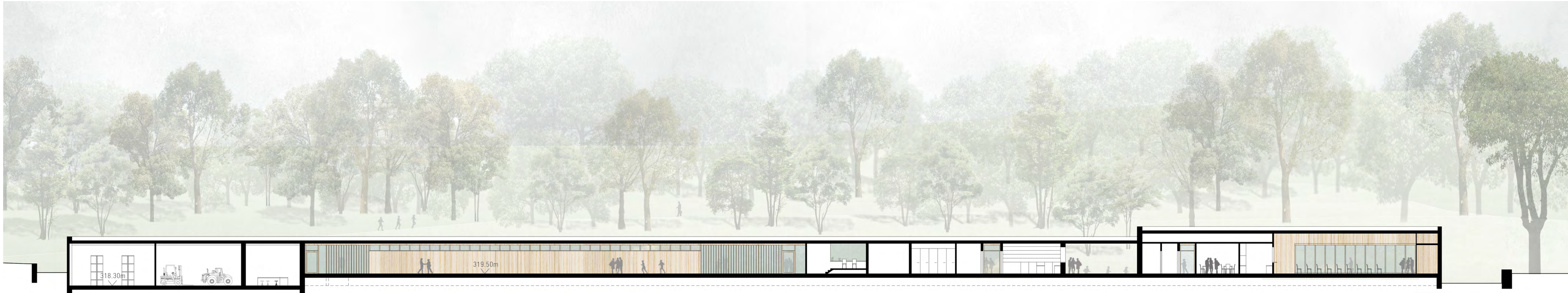
LÄNGSSCHNITT 1:200
